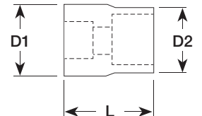
DIN 3124 / ISO 2725-1
