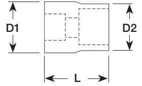
DIN 3124 / ISO 2725-1
